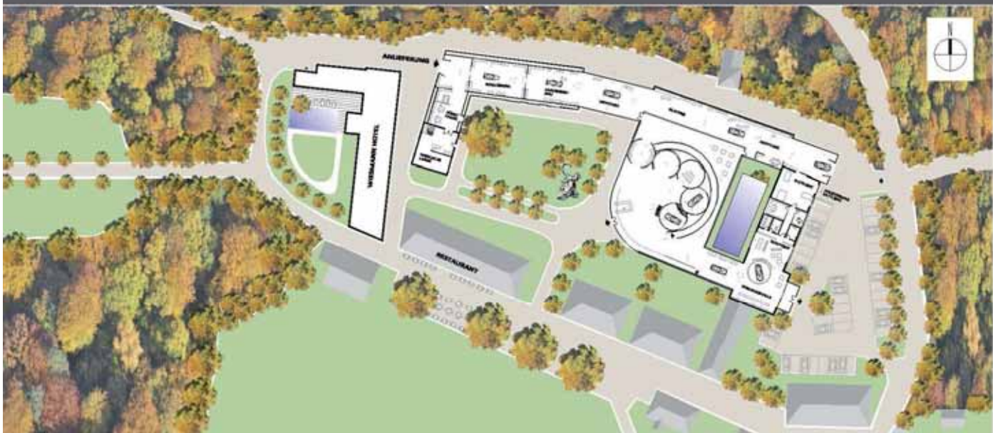
GRUNDRISS ERDGESCHOSS M 1:500
